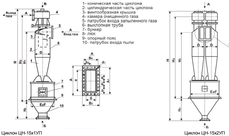
Циклон ЦН-15х1УП
